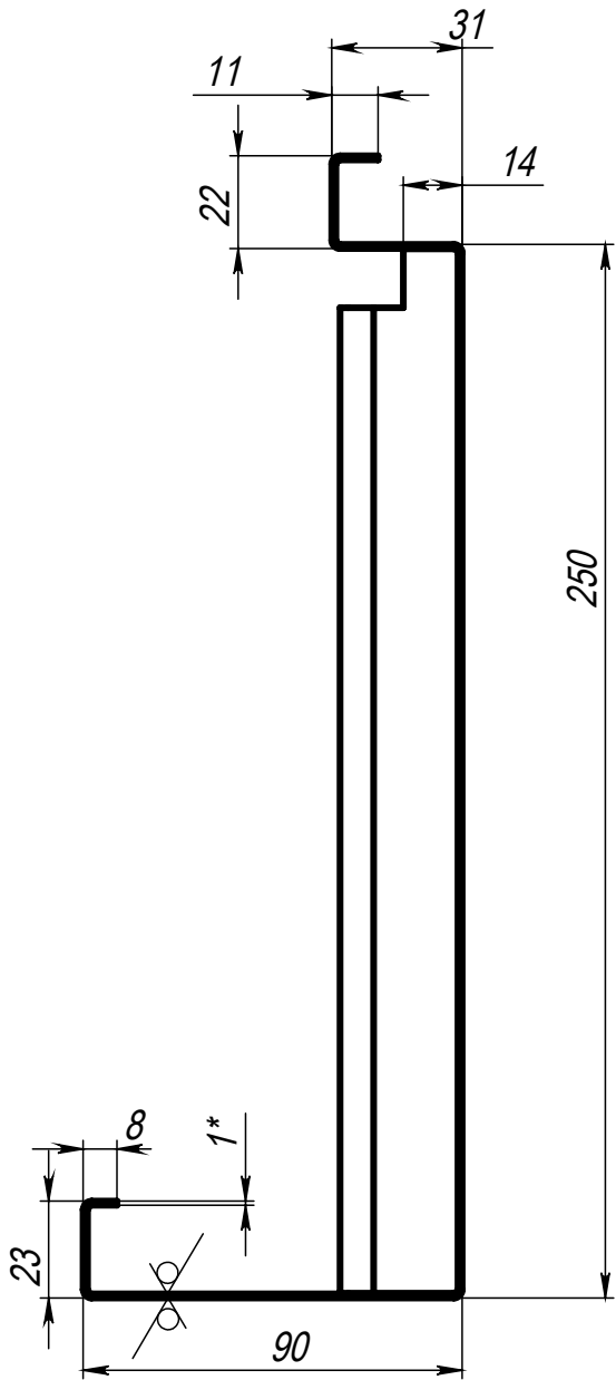
M-M (1 : 2)
